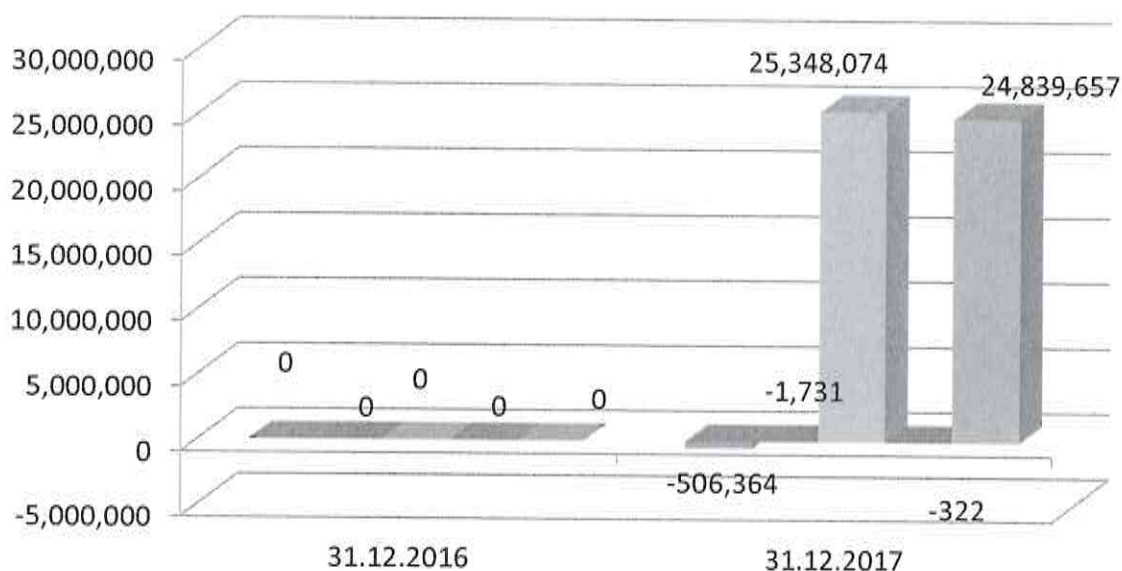
Fluxul de numerar metoda indirectă
